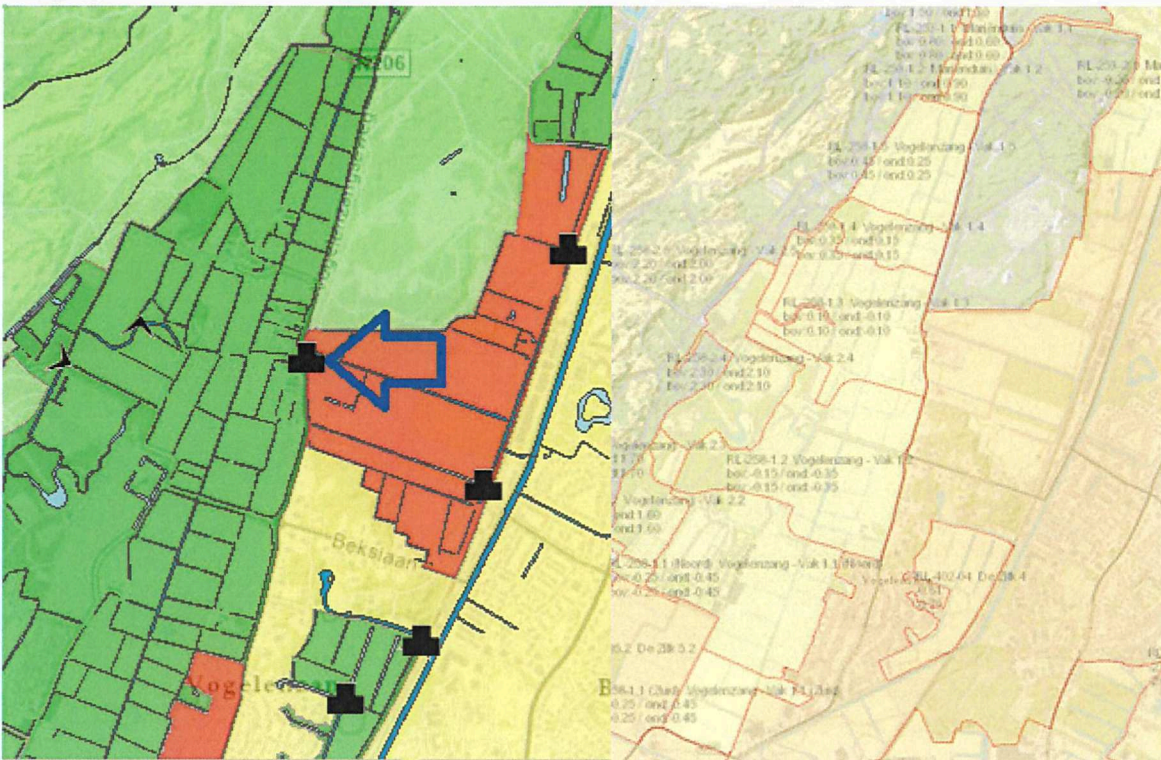
Positie gemaal
